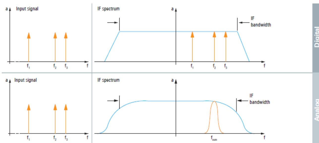
Рис. 2-2. Разрешение сигнала спектра ПЧ при цифровом и аналоговом режиме приема.
