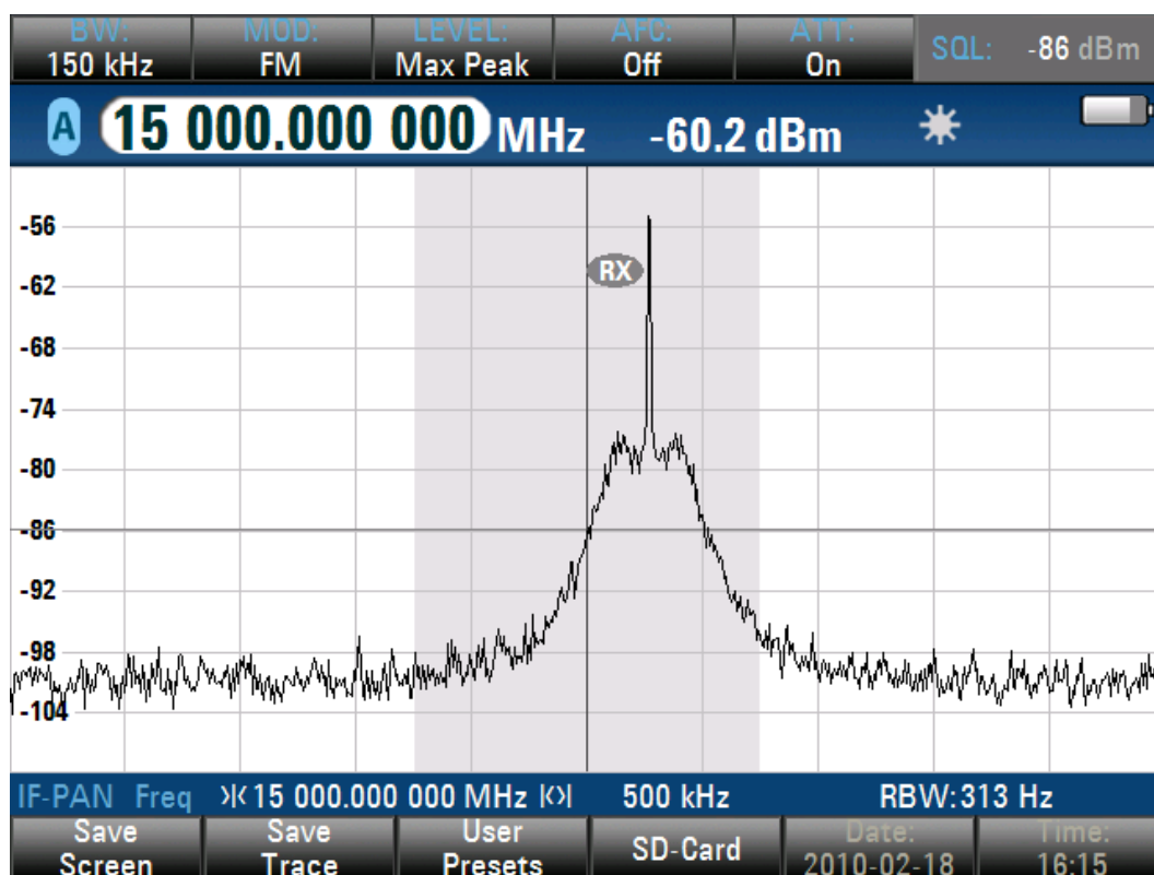
Рис. 2-5. Пример работы R&S®HF907DC с R&S®PR100
