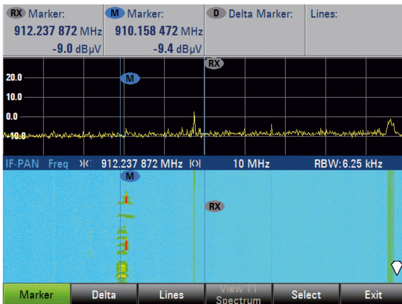
Рис. 1-3-1. R&S®PR100 обнаружение импульсных помеховых сигналов с помощью временной диаграммы
