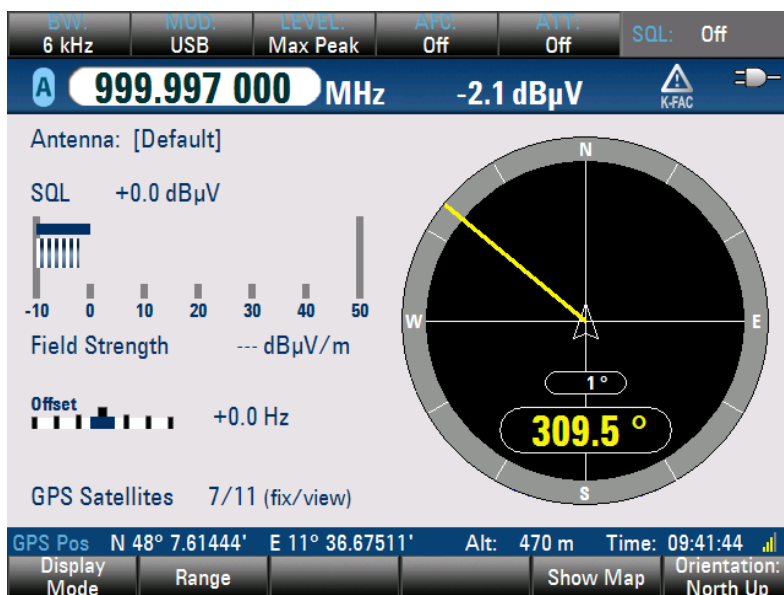
Рис. 1-8-1. Пеленгование сигналов посредством R&S®PR100 и R&S®HE400
