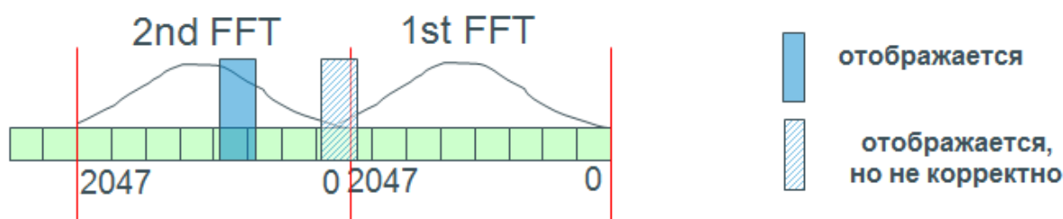
Рис. 1-2-3. Работа без потери данных
