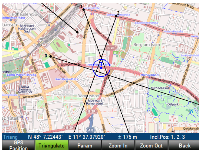
Рис. 1-8-2. Функция триангуляции, основанная на сложении результатов пеленгования
