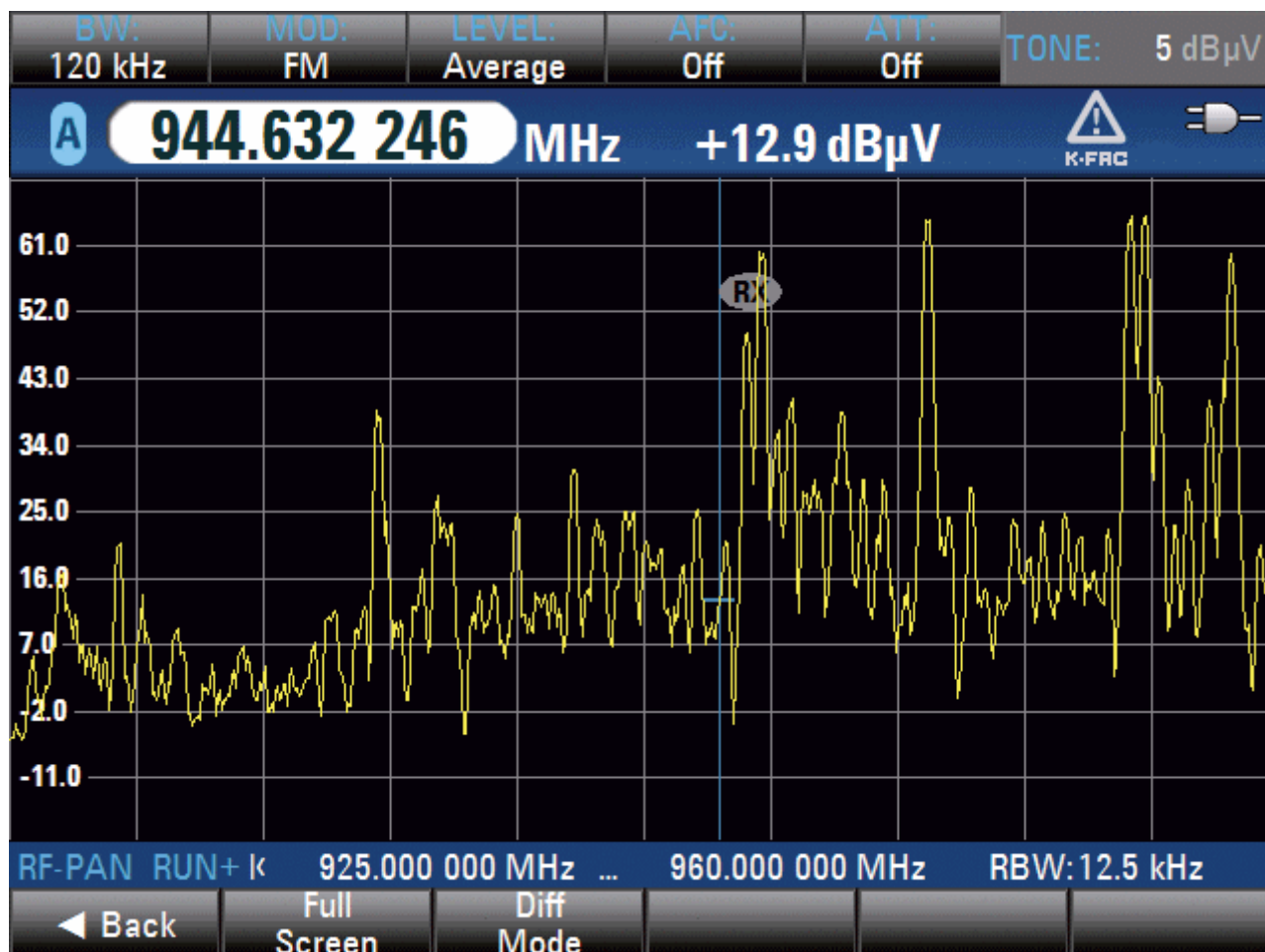
Рис. 1-3-2. Типовой спектр радиосигнала без помех
